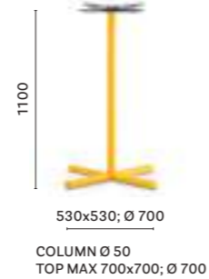
4756 Poseur table base, cast-iron base
